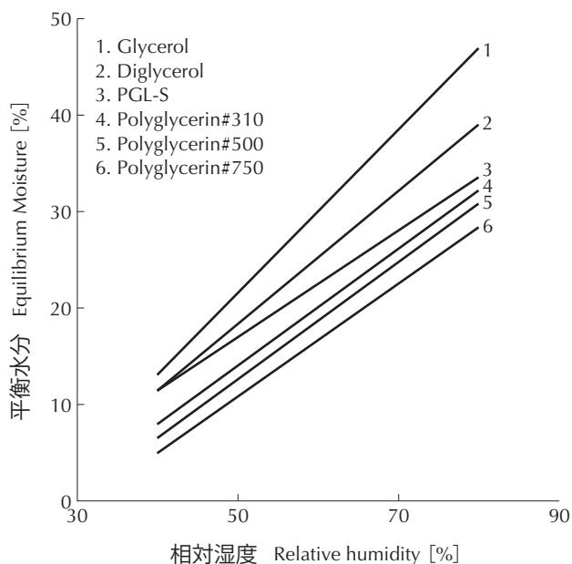
ポリグリセリン吸湿性 Hygroscopicity of Polyglycerol
