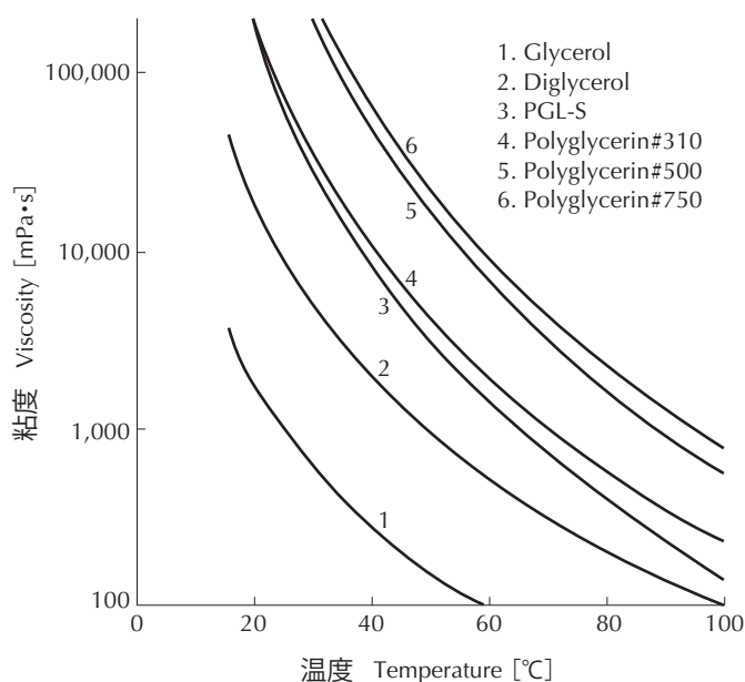
ポリグリセリンの粘度 Viscosity of Polyglycerol
